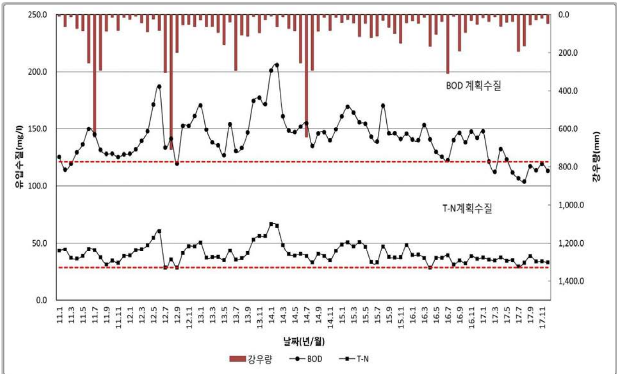
<그림 4.5-14> 최근 5년간 유입수질
