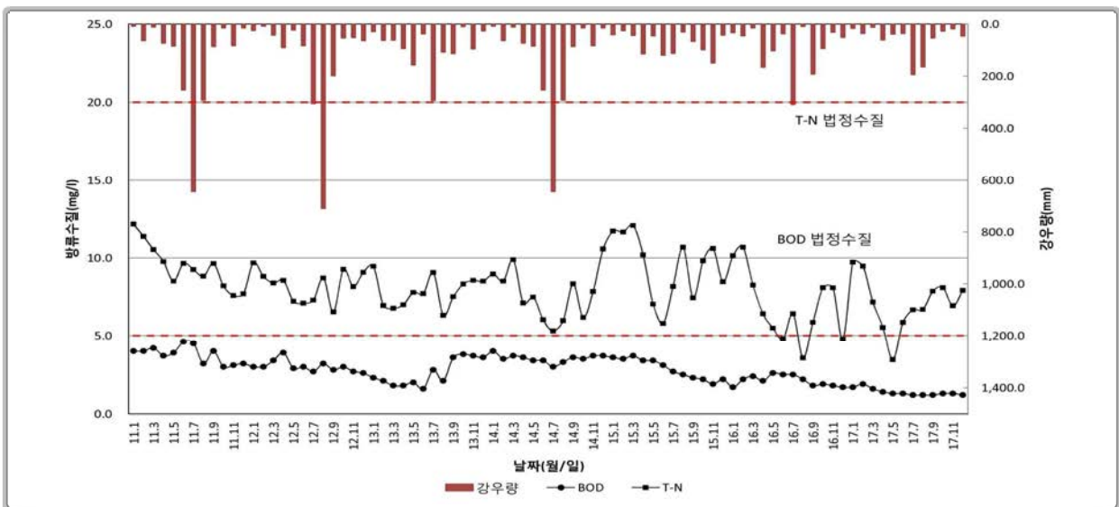
<그림 4.5-15> 최근 5년간 방류수질
