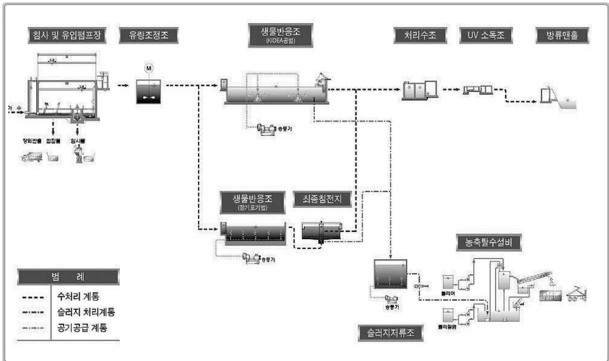
<그림 4.5-12> 서수 공공하수처리시설 처리공정도
