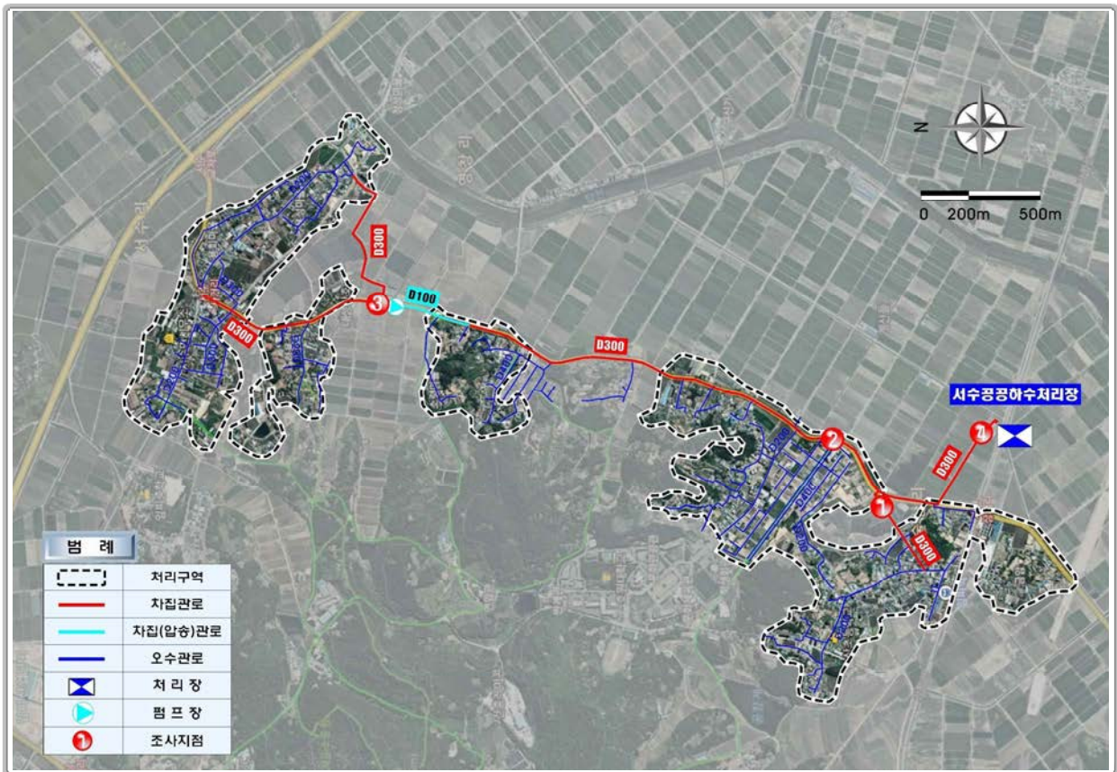
<그림 4.5-5> 서수처리구역 유량 및 수질조사
