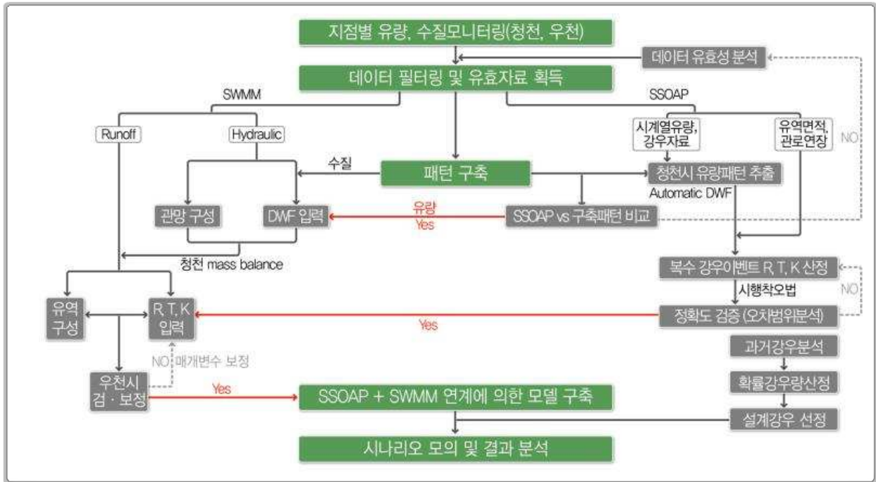
<그림 4.5-23> SSOAP과 SWMM연계에 의한 모의수행절차 모식도
