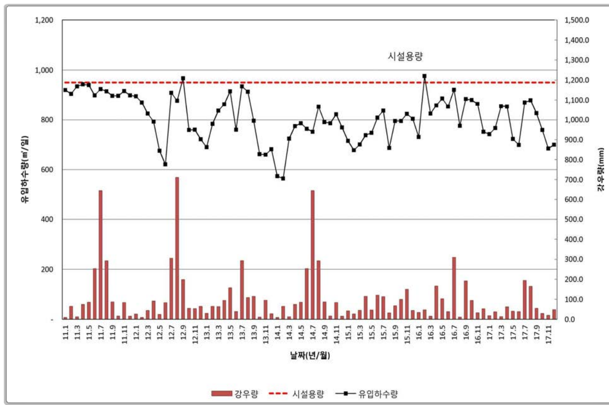
<그림 4.5-13> 최근 5년간 유입하수량
