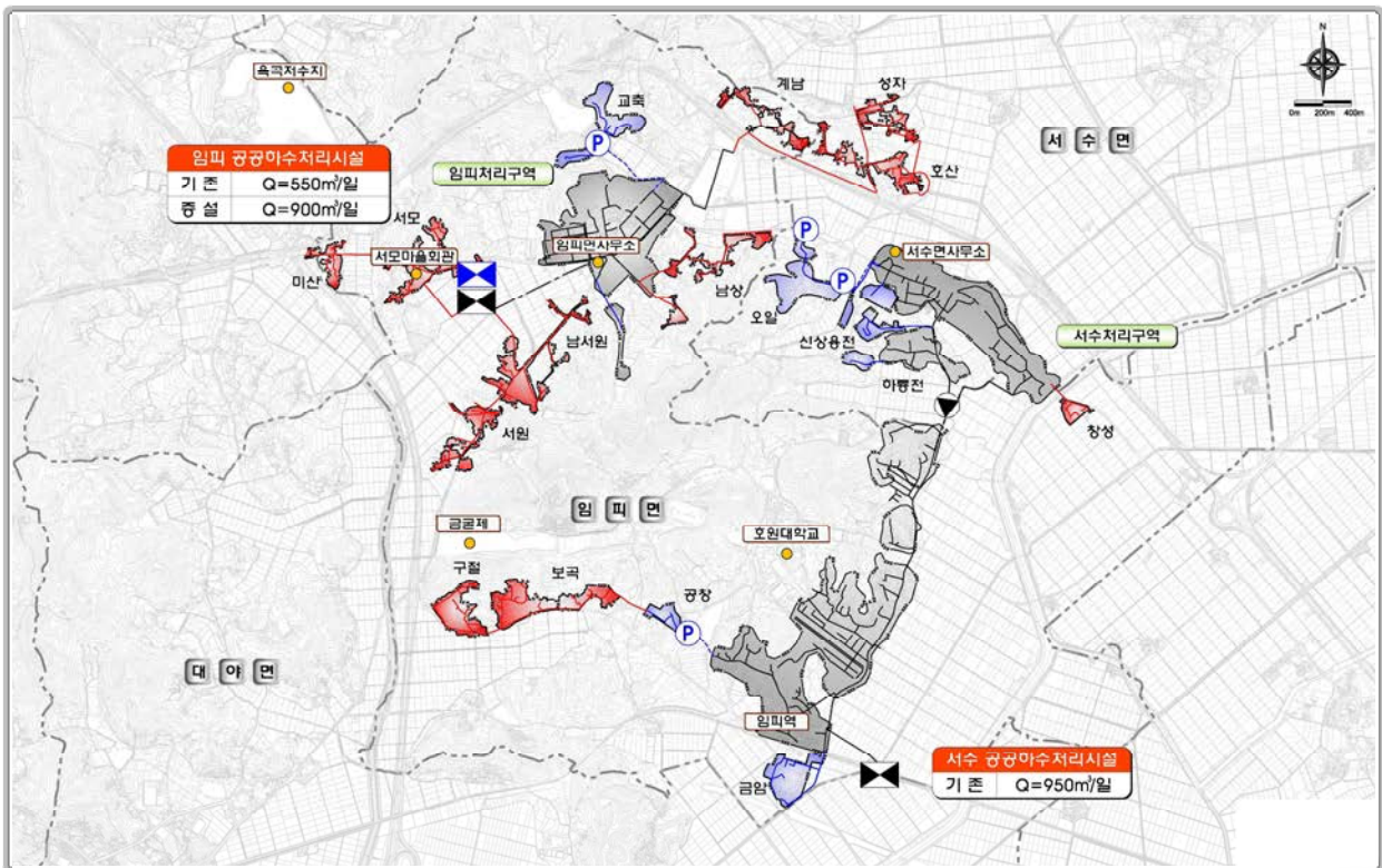
<그림 4.5-10> 신설 펌프장 위치도
