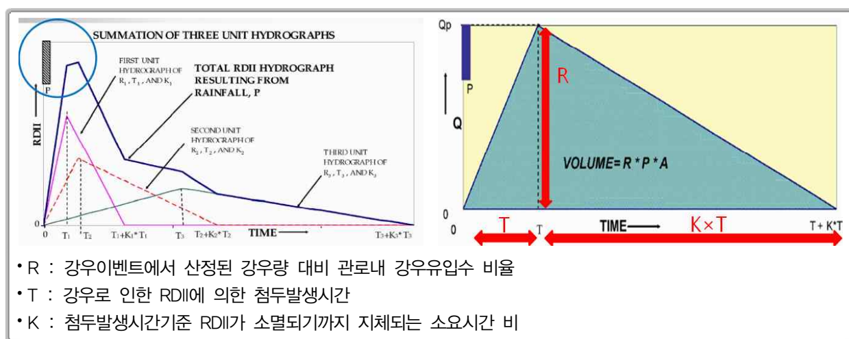
<그림 4.5-22> RTK Method 모식도
