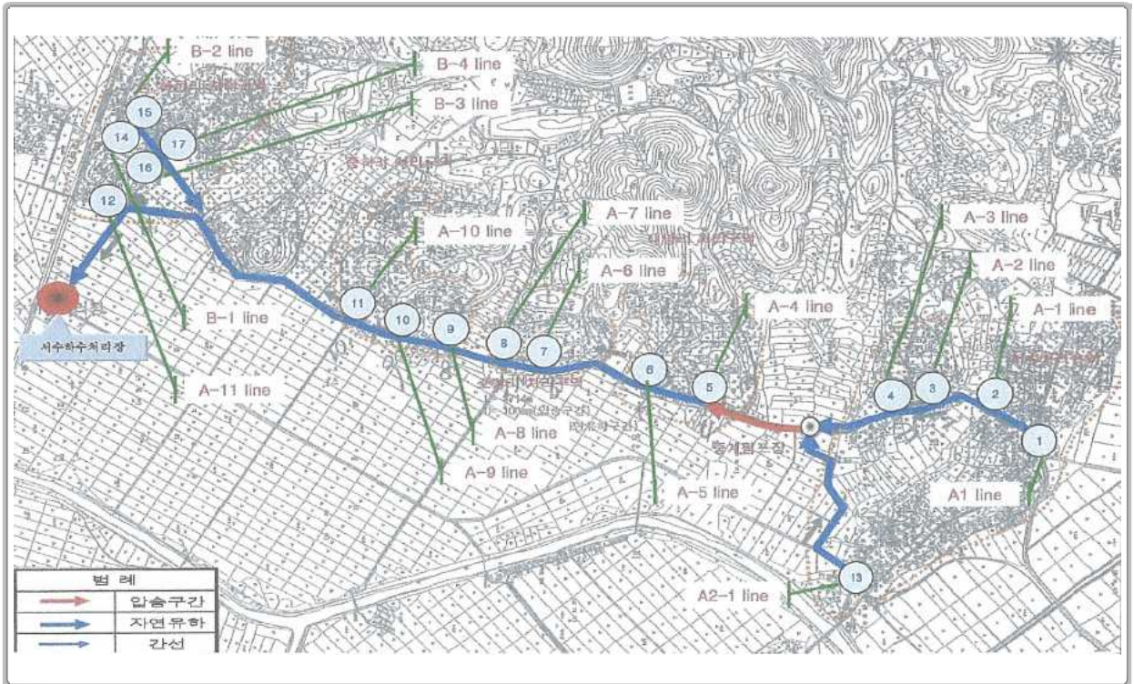
<그림 4.5-7> 관로내부조사 위치도
