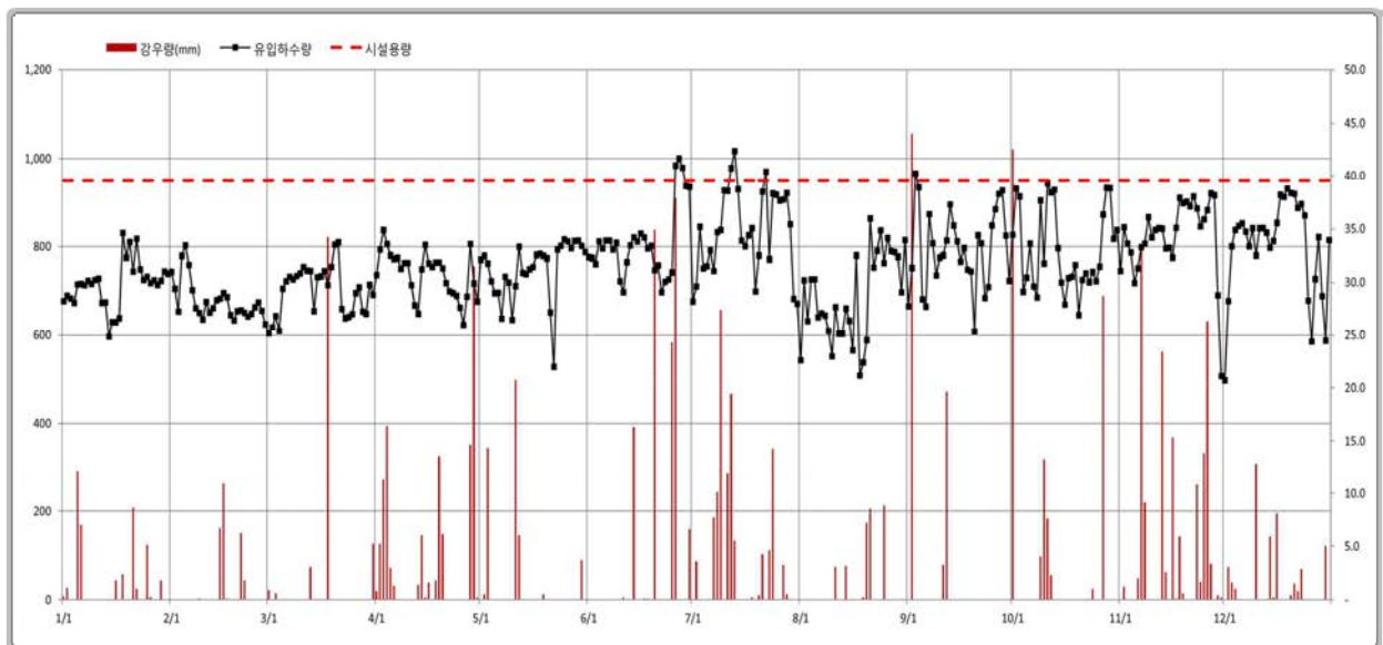
<그림 4.5-18> 강우량에 따른 하수유입 현황
