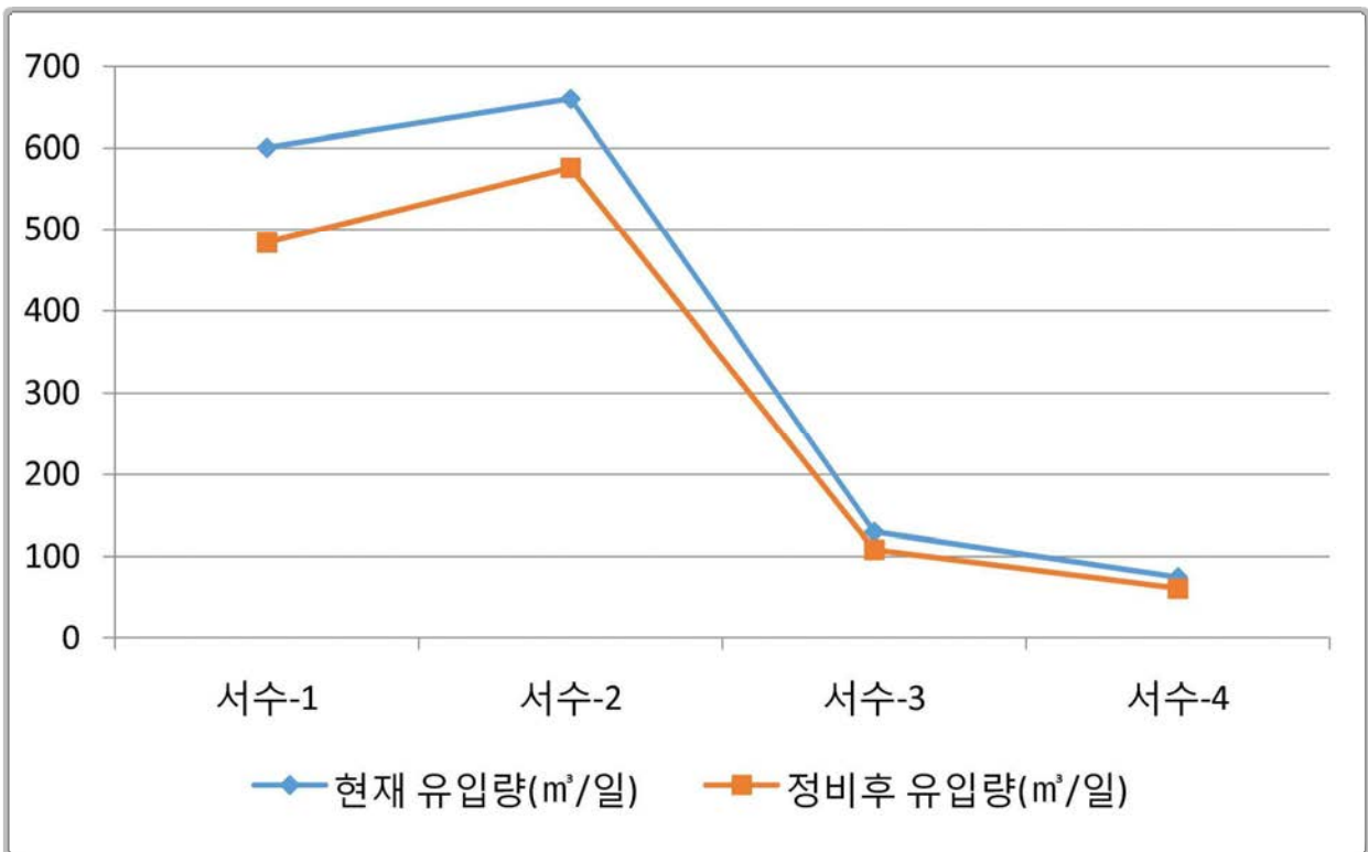
<그림 4.5-9> 오수관로 I/저감 계획
