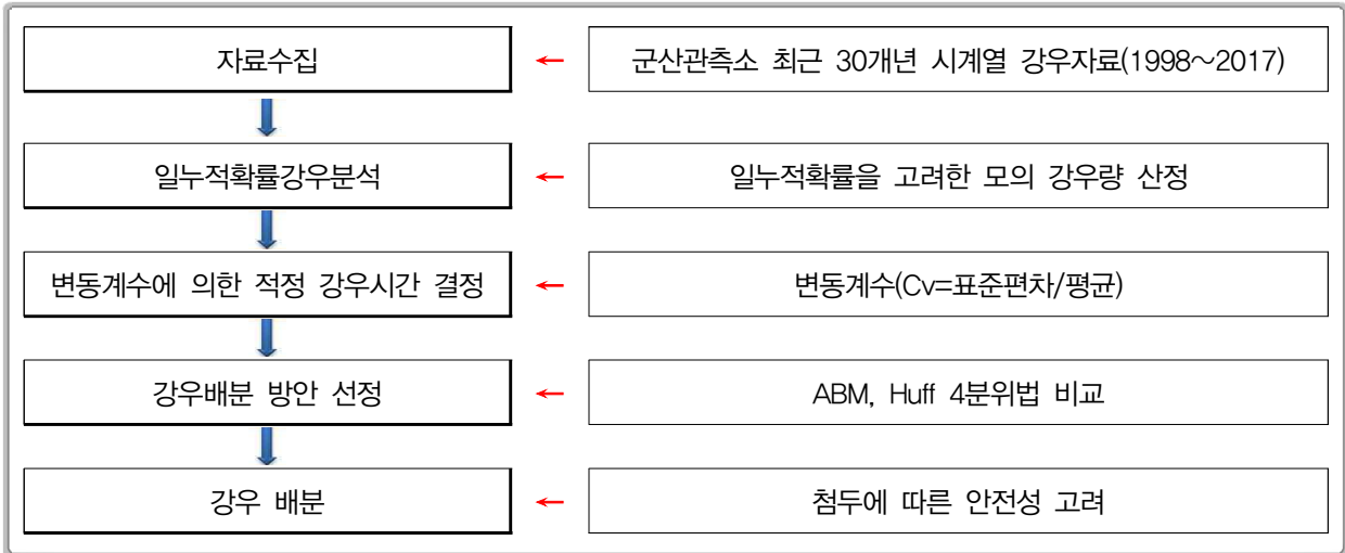
<그림 4.5-24> 설계 대상강우 분석 흐름도
