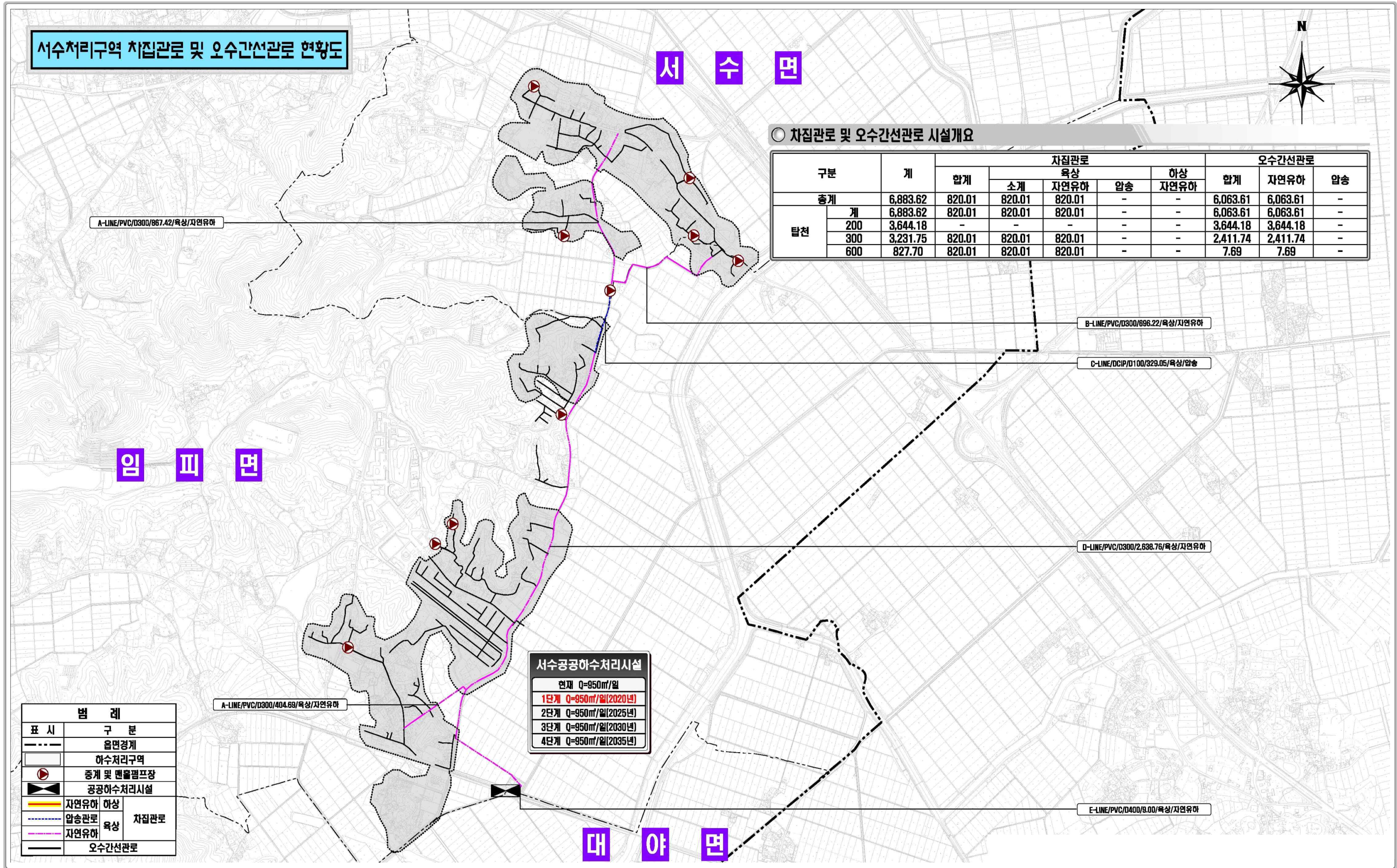
<그림 4.5-2> 서수처리구역 차집관로 및 오수간선관로 현황
