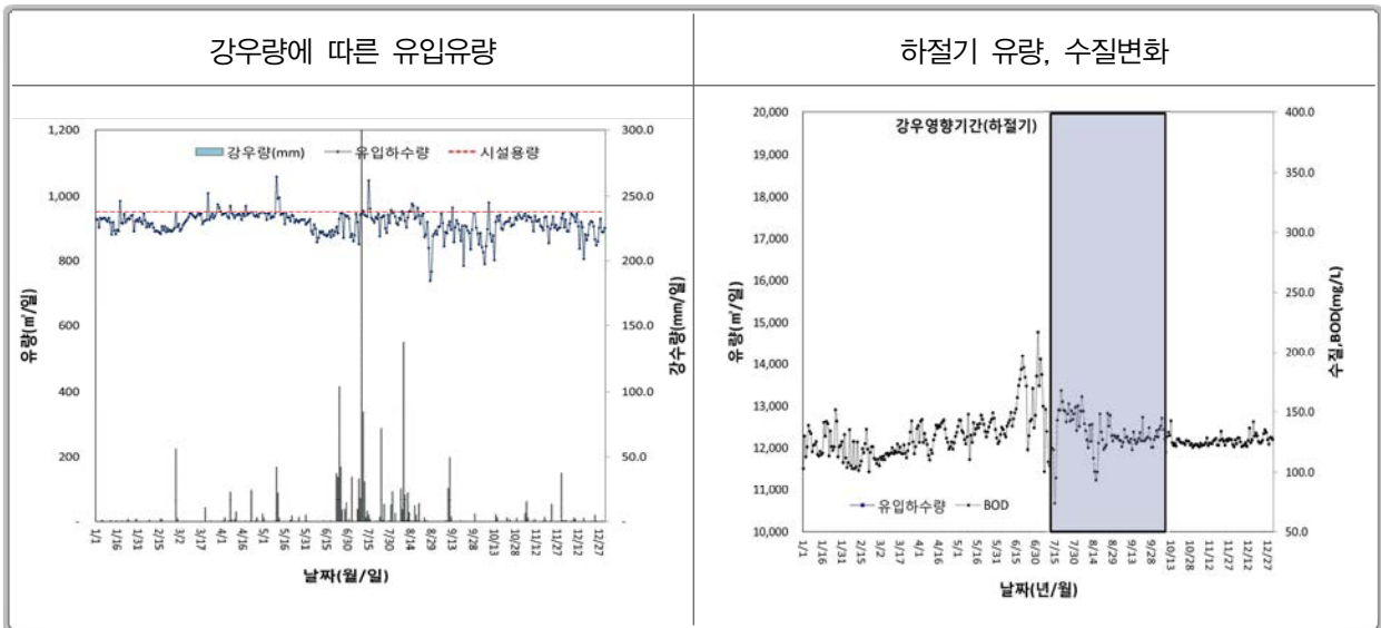
<그림 4.5-16> 하절기 유입하수량 현황(2015년)
