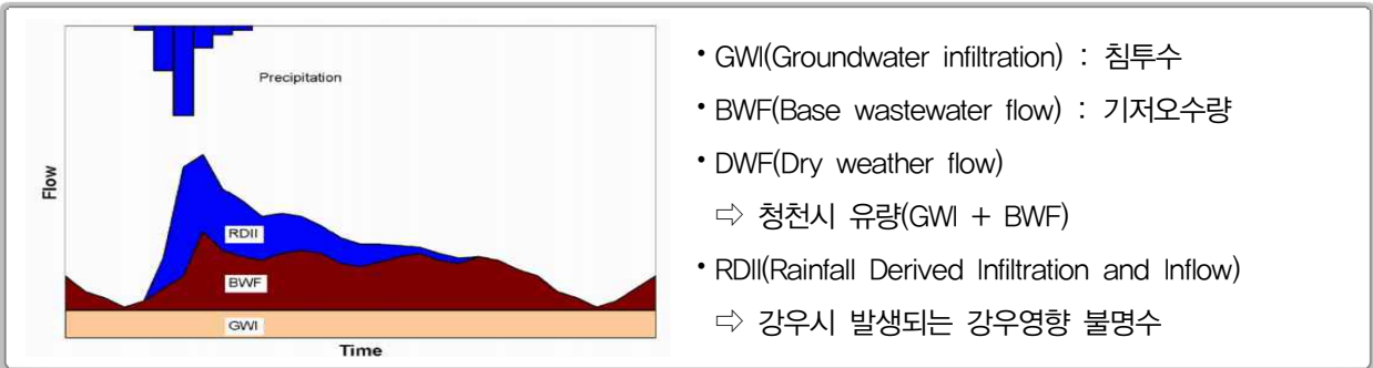
<그림 4.5-20> 강우시 하수유량 구성도
